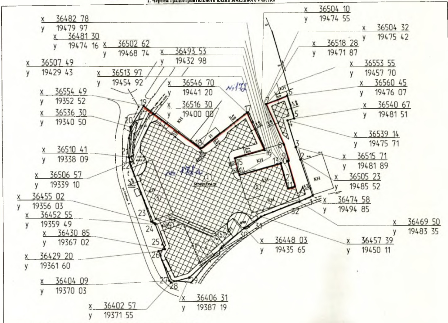
1. чертёж градостроительного плана земельного участка
